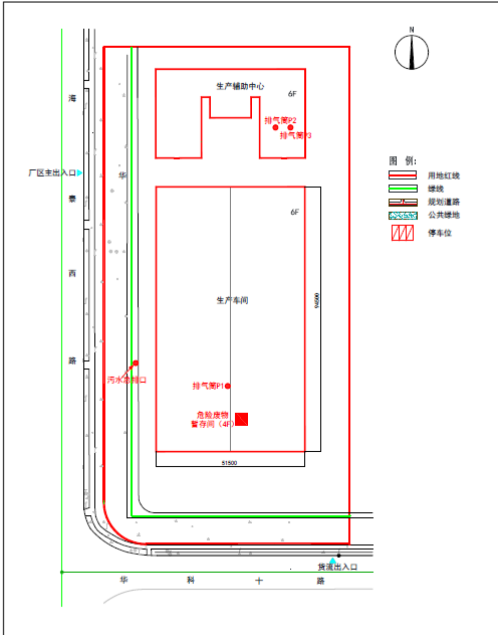
图3.2-1总平面图
