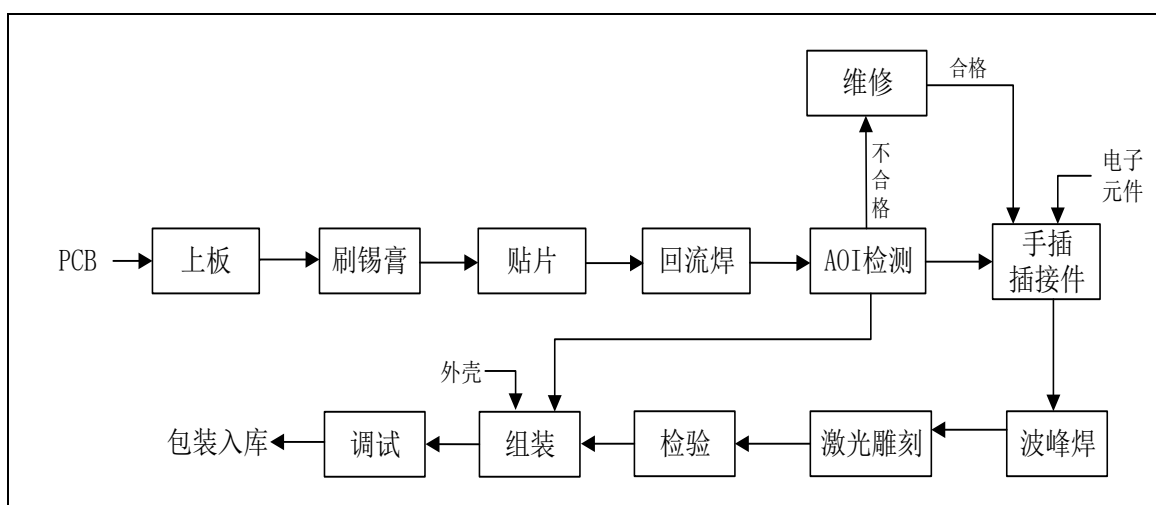
图3 天地伟业生产工艺
